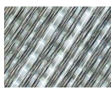
Vista della tipologia di trefolo impiegato per il rinforzo con il sistema "RETICOLATUS".
