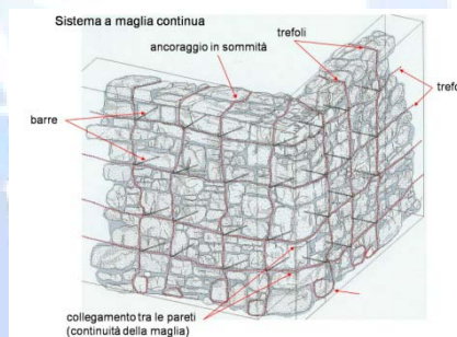
Schema di rinforzo del sistema "RETICOLATUS".
